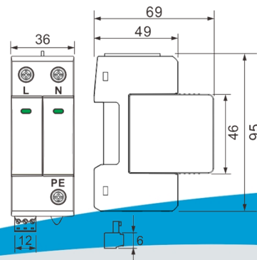
Dimensions
