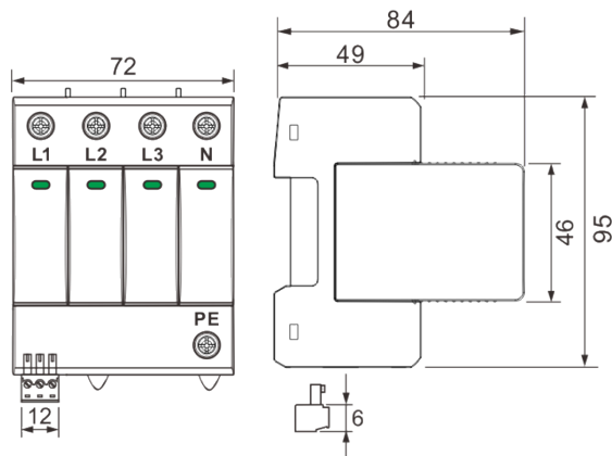
Dimensions
